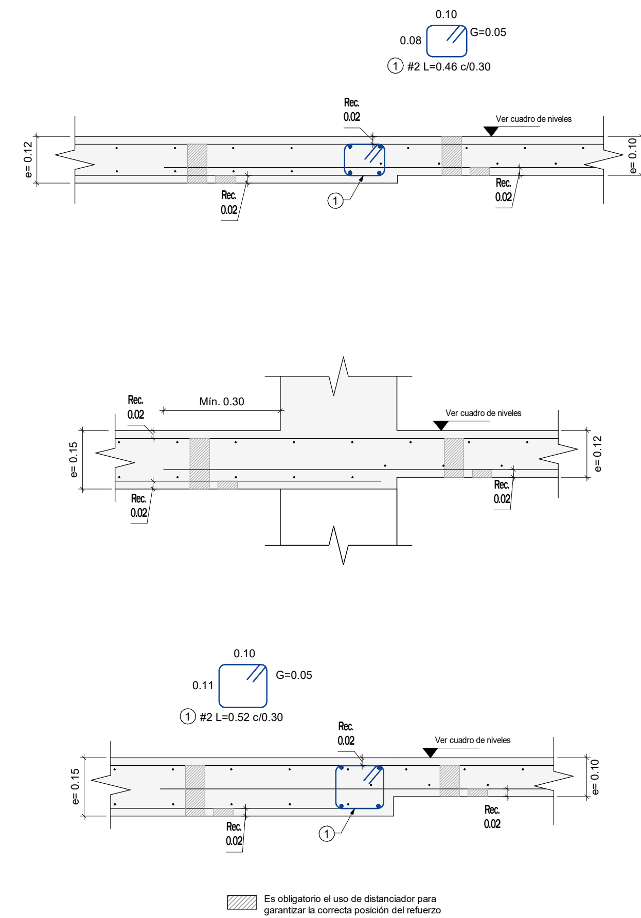
DETALLES TÍPICOS - CAMBIO DE SECCIÓN Escala 1 : 10
