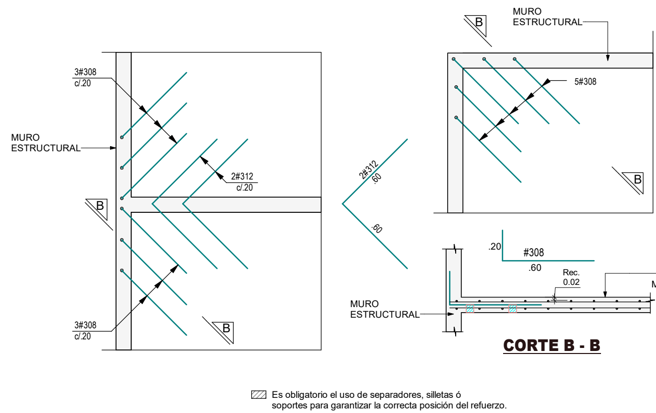
REFUERZO ADICIONAL EN PLACAS Escala 1 : 25
