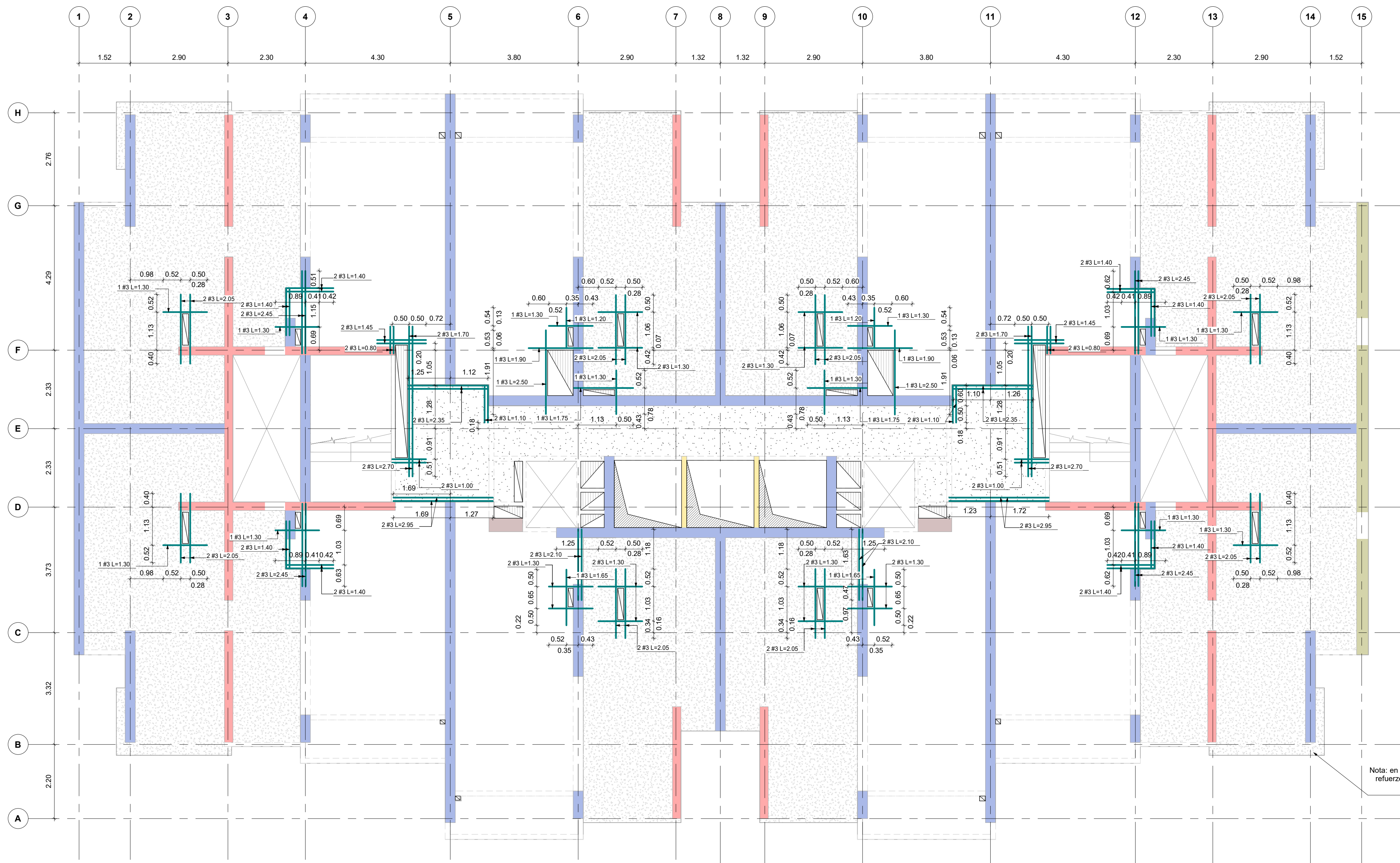
PLANTA DE REFUERZO ADICIONAL PISO TIPO 2 ( PISO 16 A PISO 22 ) Escala 1 : 75
